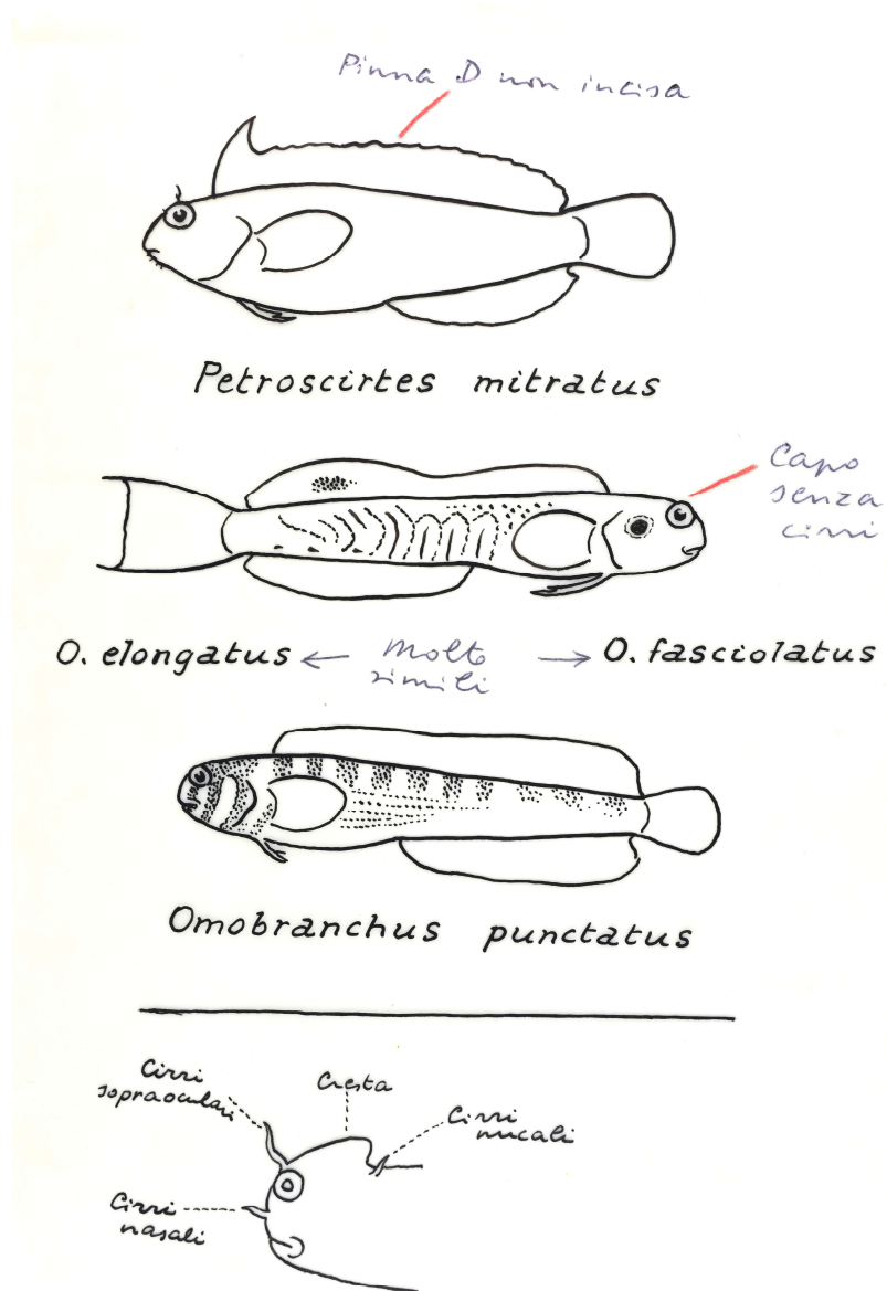
Tav. 3. Tavola originale realizzata da Enrico Tortonese, raffigurante alcuni esemplari di Blenniformi conservati nella collezione ittologica del Museo di Storia Naturale di Firenze.
